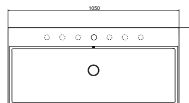
cod. ZELAVBW105 Lavabo Zenith bordo fino cm105 Zenith washbasin cm105 thin edge
