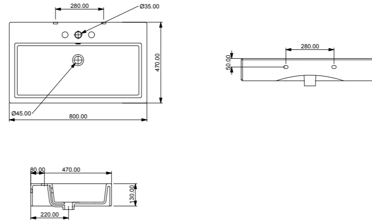
cod. QULAV80 Lavabo Quad monoforo cm. 80 appoggio o sospeso (senza foro o tre fori su richiesta) Countertop or wall-hung washbasin Quad one hole cm 80 (without hole or three holes on request)
