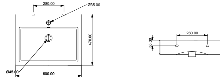
cod. QULAV60 Lavabo Quad monoforo cm. 60 appoggio o sospeso (senza foro o tre fori su richiesta) Countertop or wall-hung washbasin Quad one hole cm 60 (without hole or three holes on request)
