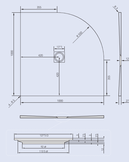
MISURE TECNICHE MODELLO ANGOLARE 100X100 CM
