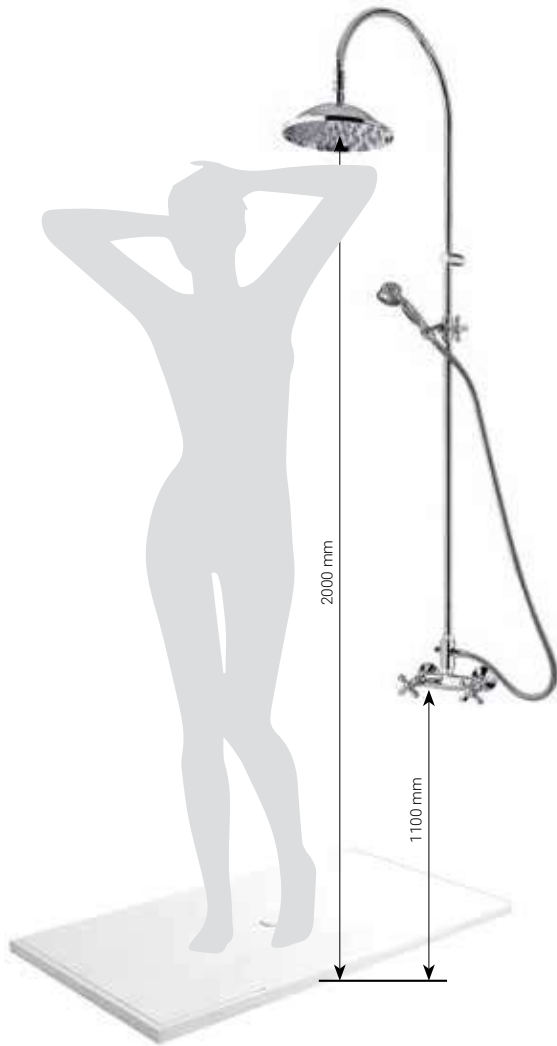
DOCCIA SHOWER
