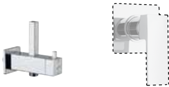
Preso acqua per installazione con monocomando o termostato a incasso già esistente (non fornito). Water supply for installation with concealed shower mixer. Mixer not included.
