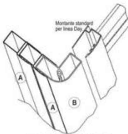
Esempio assemblaggio dei profili A, B.
