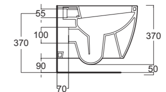
Art. 0650 Vaso Soho sospeso Soho wall hung wc bowl
