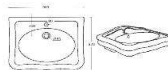
Art. 0860 Consolle sospesa o da appoggio monoforo cm 90 Wall-hung or over-counter one-hole console 90 cm
