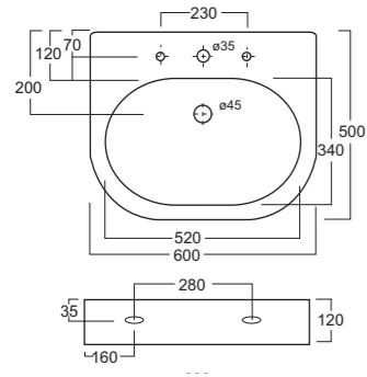
Art. 0852 Lavabo Broadway cm.60 Broadway washbasin cm.60
