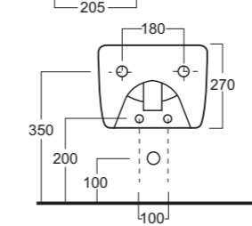
Art. 0751 Bidet sospeso Piccadilly Piccadilly wall hung bidet bowl
