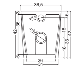
Art. 0152 Vaso Broadway Broadway wc
