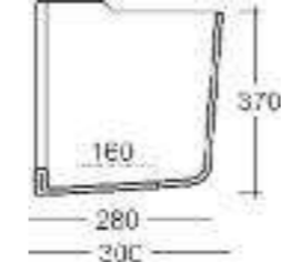
Art. 0850 Lavabo Soho cm.67 Soho washbasin cm.67
