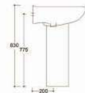
Art. 0857 Lavabo Cleo cm.67 Cleo washbasin cm.67
