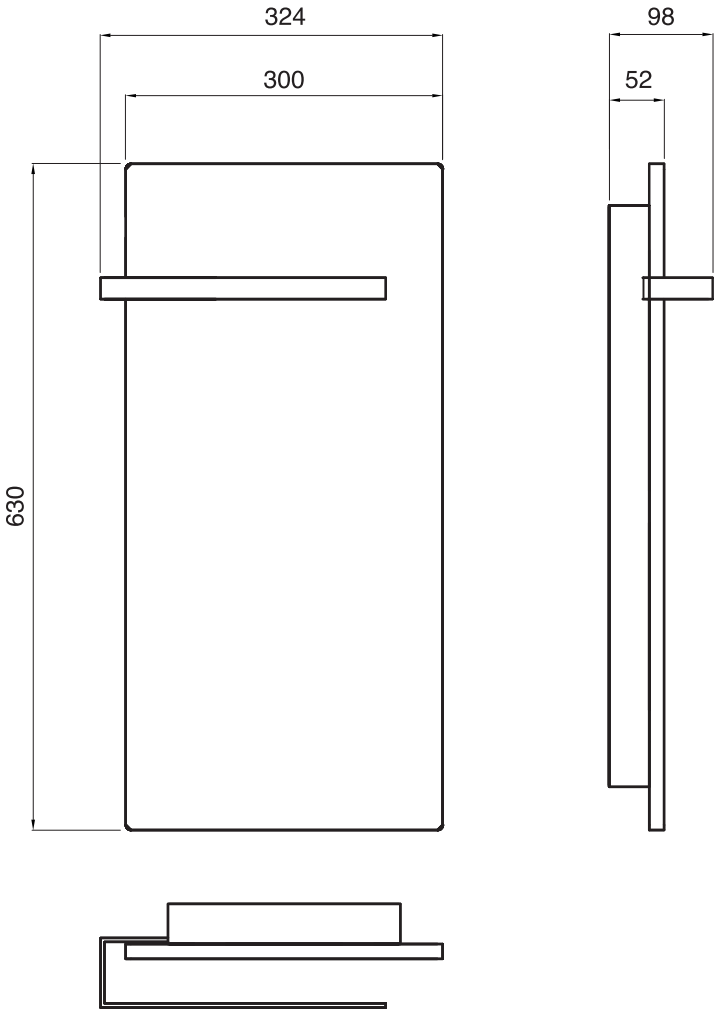
Supporto porta asciugamano in Acciaio spazzolato. Towel rail in brushed steel.
