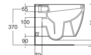
Art. 0650 Vaso Soho sospeso Soho wall hung wc bowl
