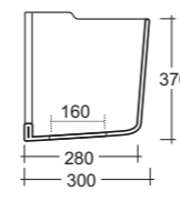
Art. 0850 Lavabo Soho cm.67 Soho washbasin cm.67 Art. 0950 Semicolonna Soho Soho semi-pedestal
