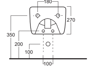
Art. 0751 Bidet sospeso Piccadilly Piccadilly wall hung bidet bowl
