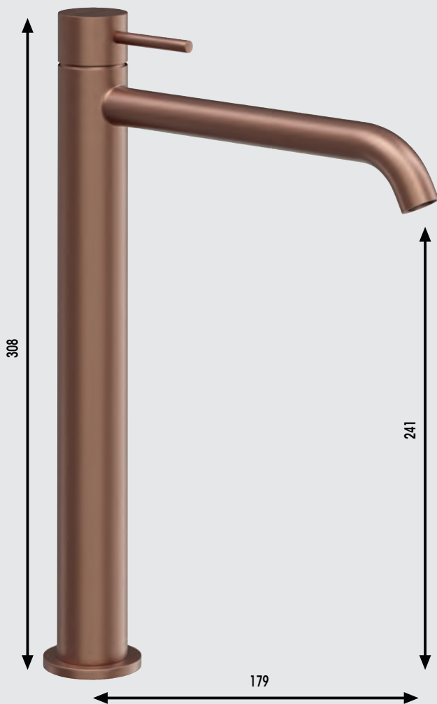
cod. RUB225 LIFE Ø34 - Lavabo d'arredo
